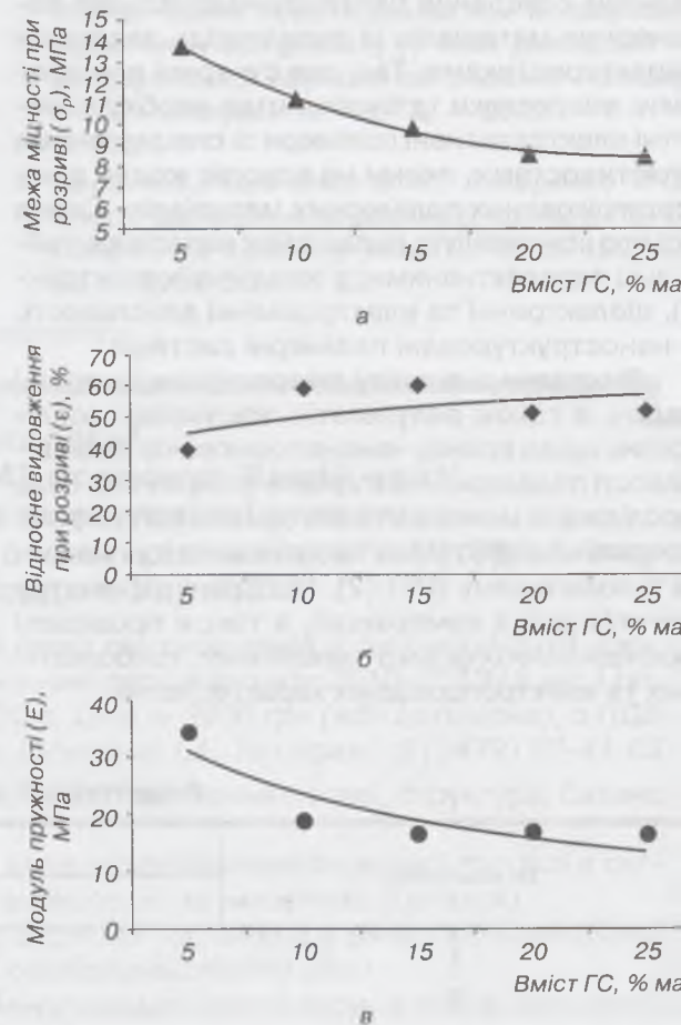
Рис. 2. Залежність властивостей ПЕ композиції від вмісту ГС: а — межа міцності при розриві; б — відносне видовження при розриві; в — модуль пружності
