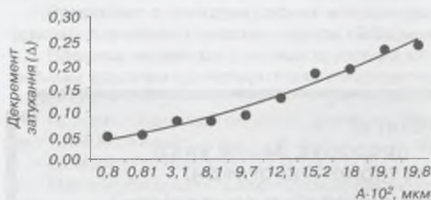
Рис. 4. Амплітудна залежність декременту затування ПЕ композиції, наповненої 20% мас. ГС
