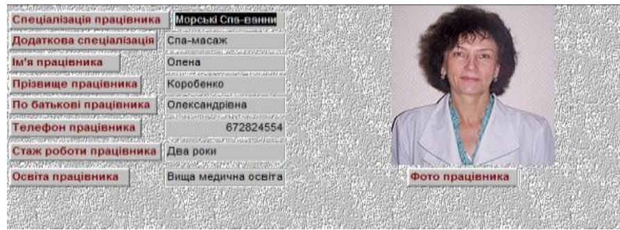
Рис.5. Характеристика персоналу
