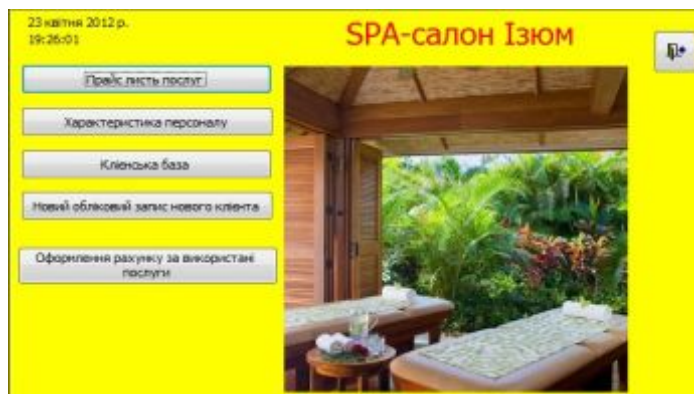
Рис.3. Головна форма
