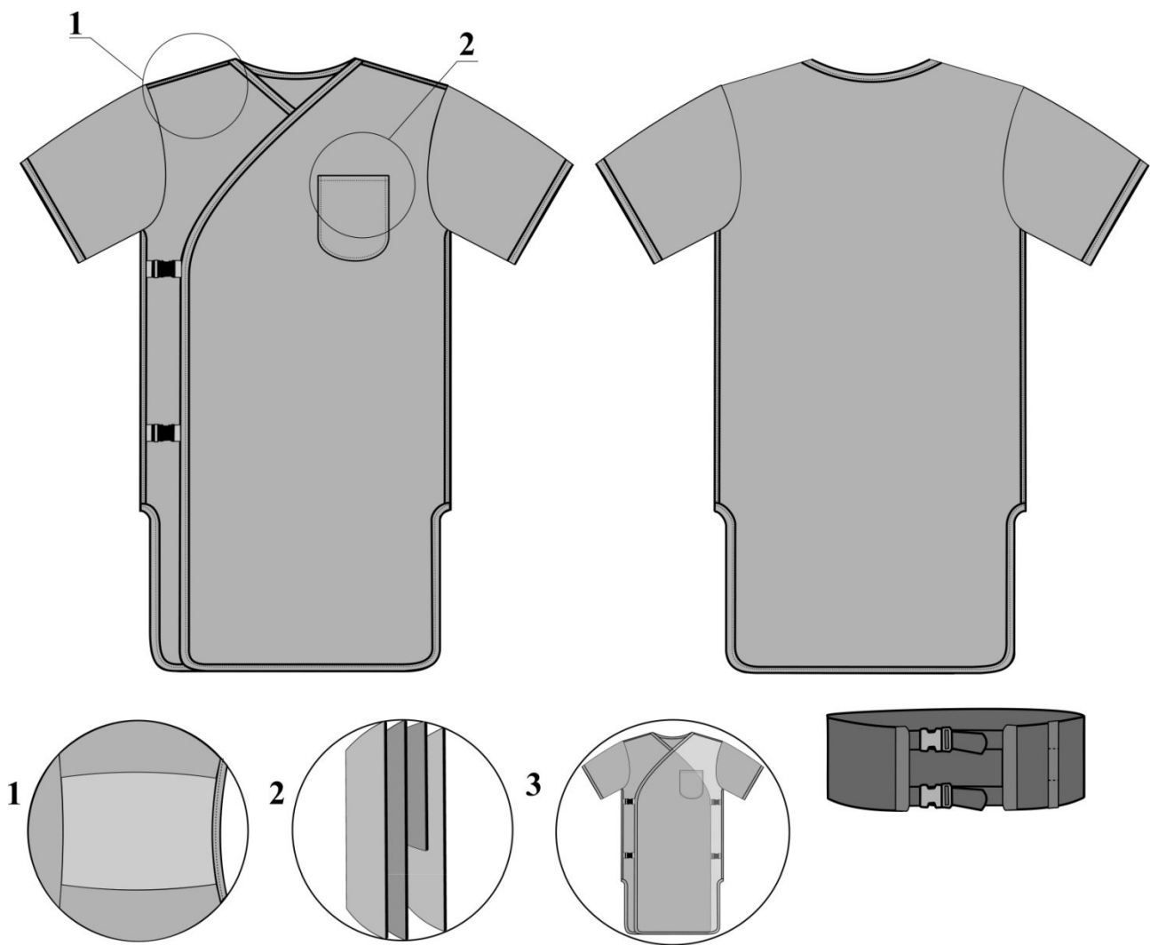
Рисунок 1 – Зовнішній вигляд запропонованої моделі халата для захисту від рентгенівського випромінювання: 1 - схема внутрішнього боку халата в ділянці плечового шва де розташовані поролонові плечові накладки; 2- схема розташування шарів матеріалів спереду зверху на ділянках, де пілочки не перекривають одна одну (двох шарів свинцевмісткого вінілового рентгенозахисного матеріалу); 3- схема розташування двох додаткових застібок-фастекс для підтримки нижньої пілочки;. 4- зображення поясу з широкої еластичної тасьми.
