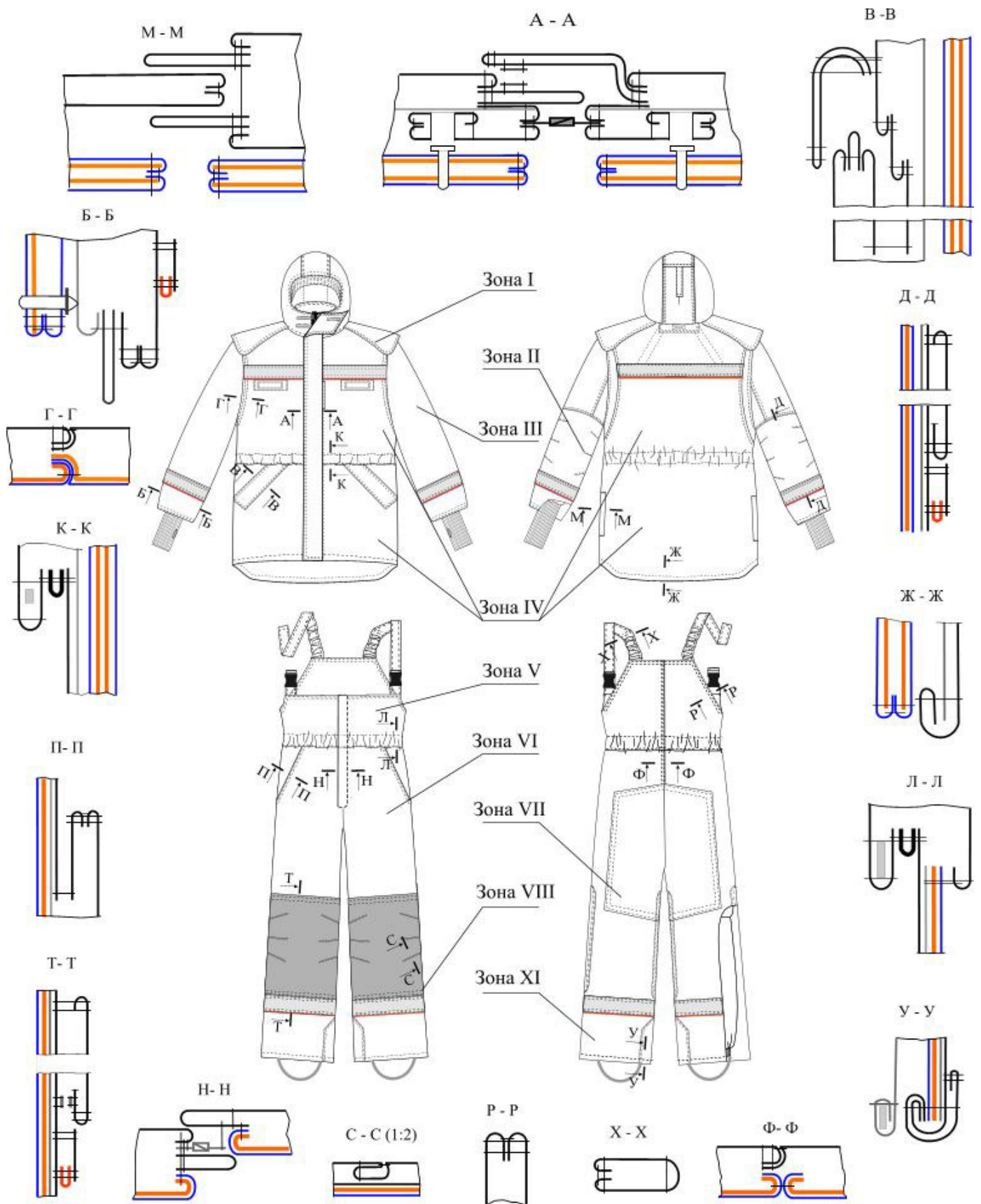
Рис. Конструктивно-технологічне рішення комплекту аварійно-рятувального спеціального одягу «ТАРК – 12» та схеми обробки основних вузлі із зональним розташуванням пакетів
