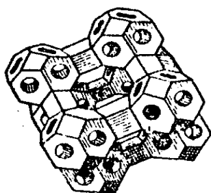
Рис.2. Каркасна структура кристалу цеоліту
