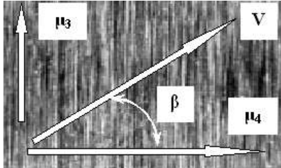
Рис.1. Анізотропія фрикційних властивостей напрямної
