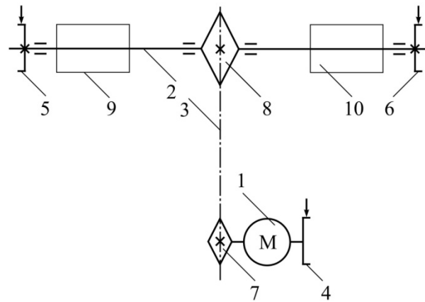
Рис. 1. Кінематична схема приводу основов'язальної машини:
